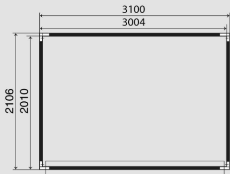
PLANTA
