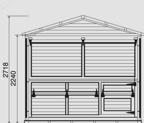
ALZADO
