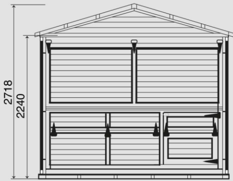
ALZADO
